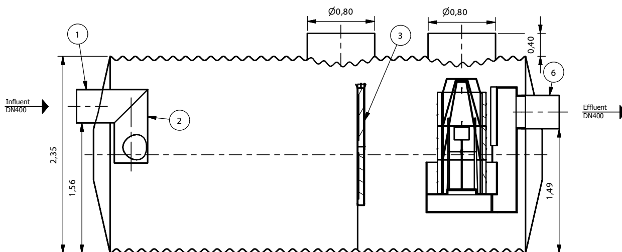
A-A ( 1 : 40 )
