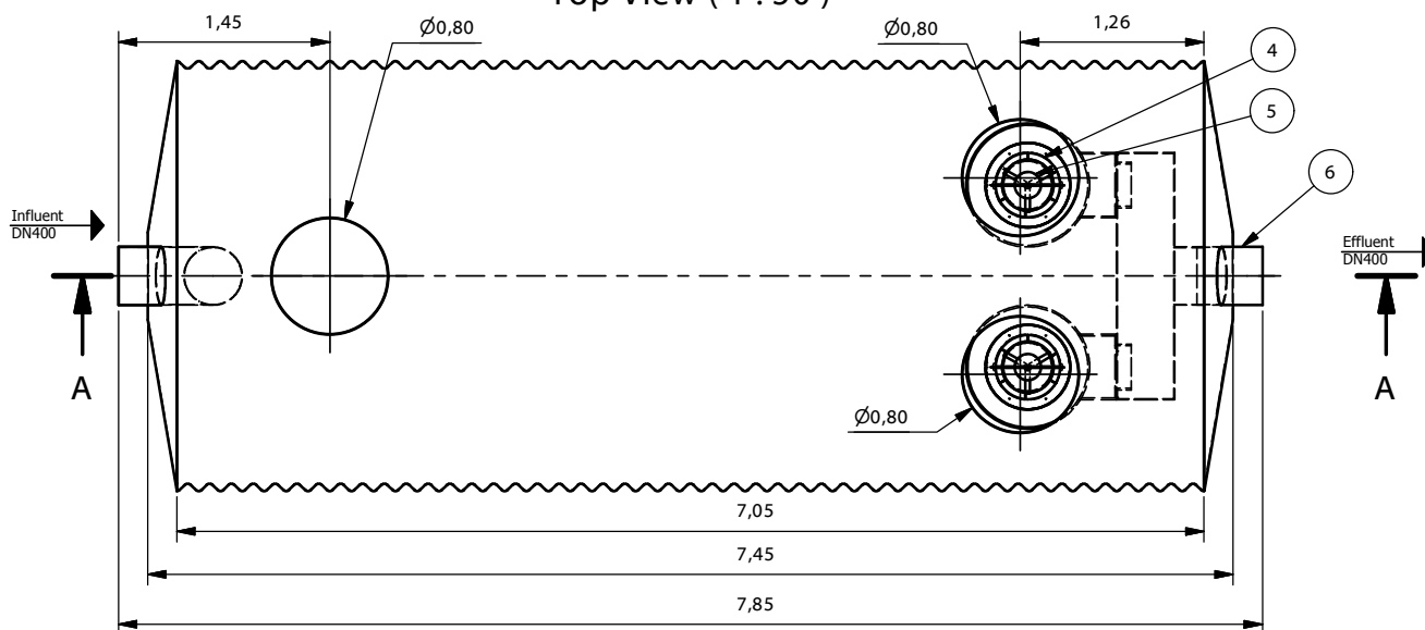
TNS 200-5-A ( 1 : 125 )
