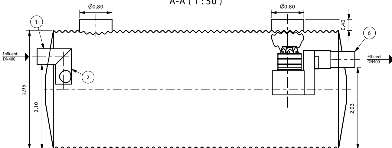
A-A ( 1 : 50 )
