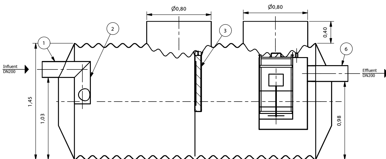
A-A ( 1 : 25 )
