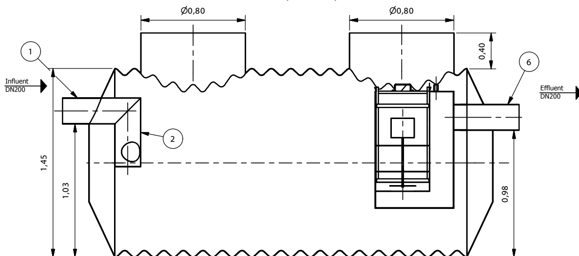
A-A ( 1 : 25 )
