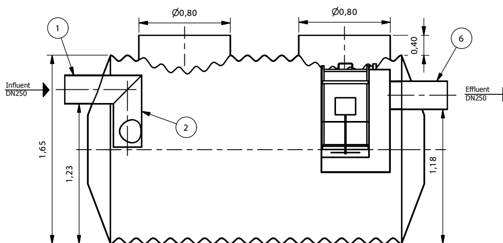
A-A ( 1 : 30 )
